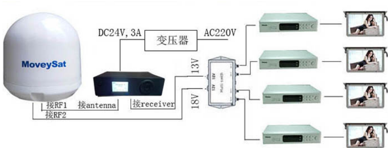
多机接线图
