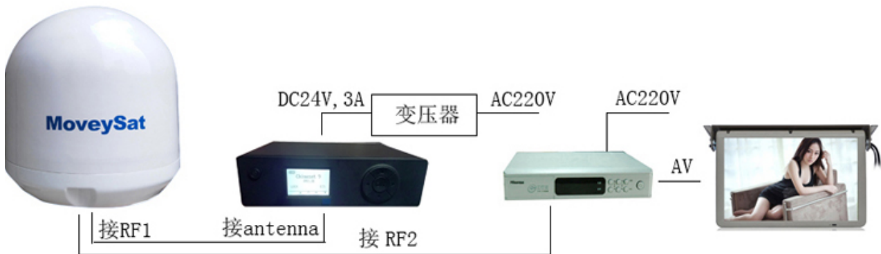
多机接线图
